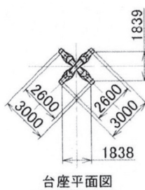
台座平面図
