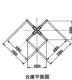
台座平面図
