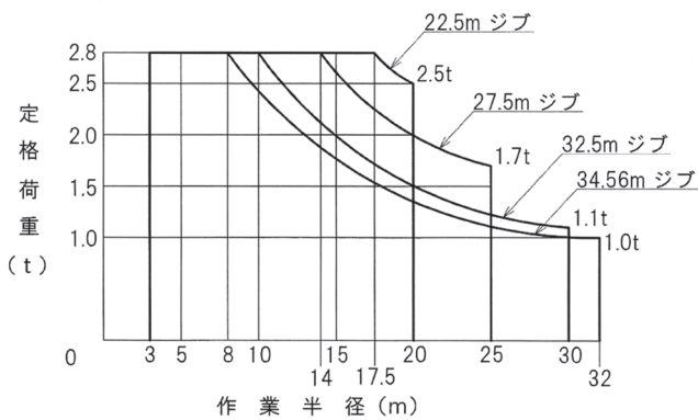
定格荷重線図
