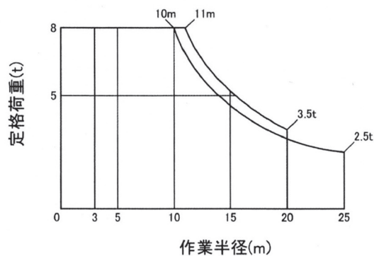
定格荷重線図
