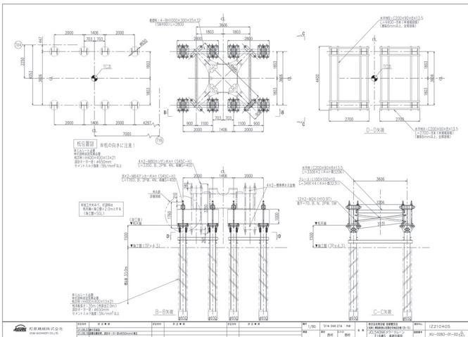
基礎図
