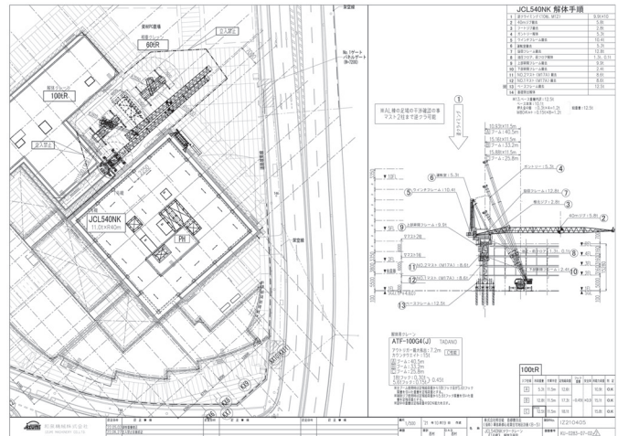
解体計画(本体立面)
