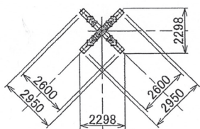
台座平面図 (アタッチメント無)
